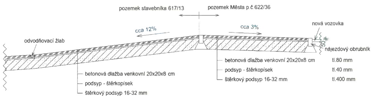
Řez M 1:25 - sjezd z pozemku p.č.622/36 na p.č.617/13, k.ú. Pohledec
